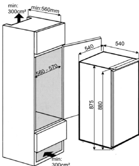
Einbauskizze
